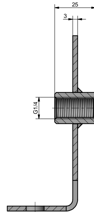
A-A (1:1)
