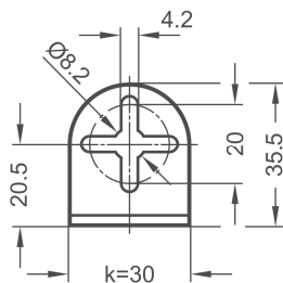
Lug width k=30
