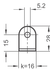
Lug width k=16
